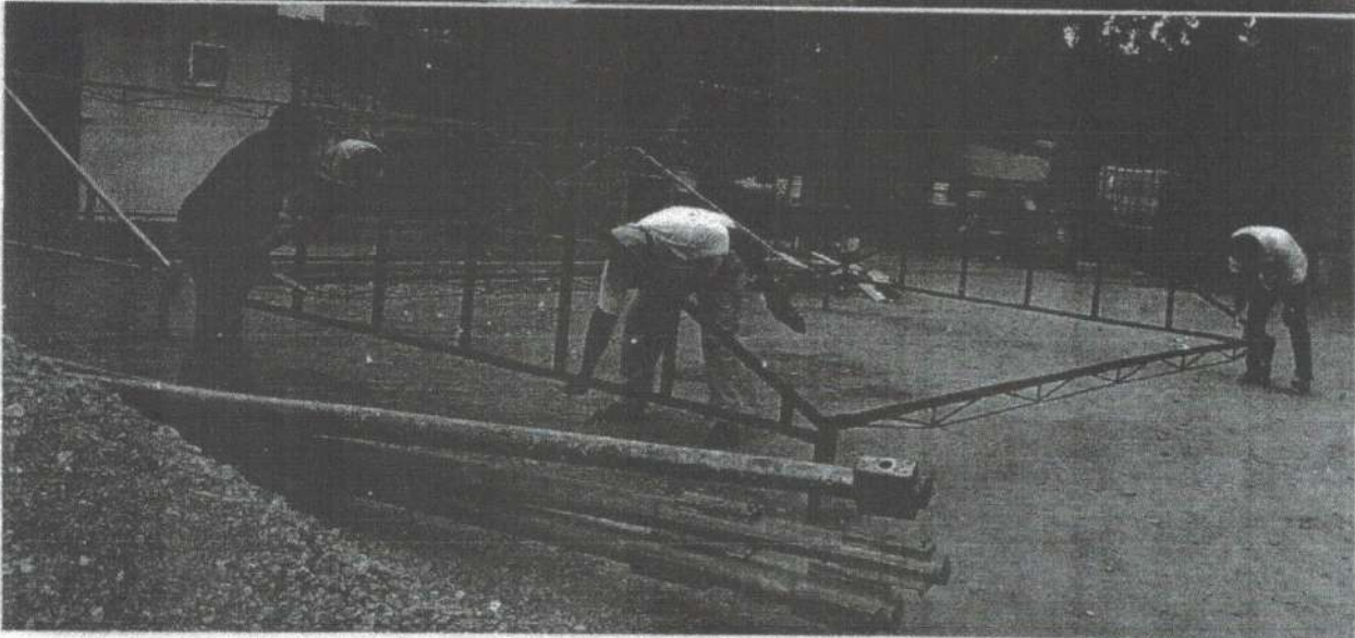
ELABORACION DE ESTRUCTURAS PARA TOLDOS PARA EL DEPARTAMENTOS DE KIOSCOS Y YARIMAS
